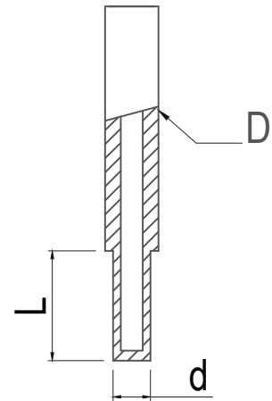
Stepped Tip Adımlı / İnceltmiş uç
